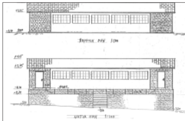
Εικόνα 2: Όψεις Κτηρίου - Ψηφιακό Κέντρο Ιστορικής Μνήμης
